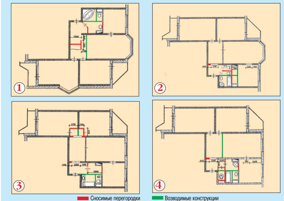
Сносимые перегородки Возводимые конструкции
