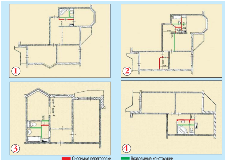
Сносимые перегородки (красная линия) Возводимые конструкции (зеленая линия)
