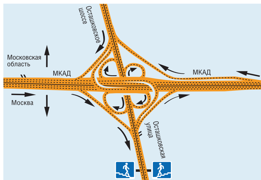
Ожидается, что пропускная способность развязки после окончания реконструкции возрастёт на 25-30%
