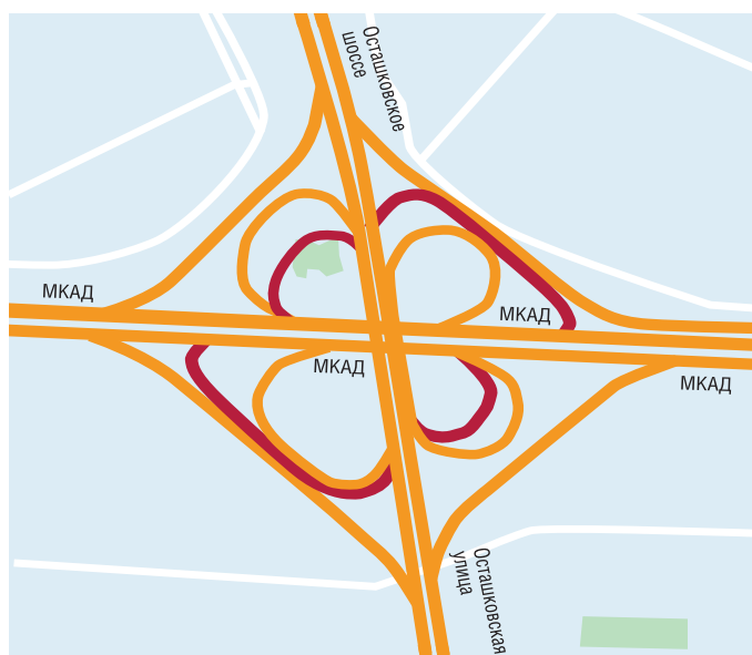
Красным выделена временная форма «клевера» на развязке, которая будет действовать во время первого этапа реконструкции. На всех временных петлях будет по одной полосе
